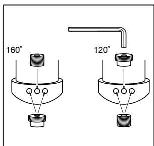
Kuva 3A
