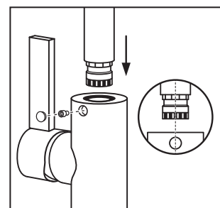
Kuva 3B4
